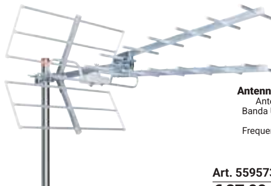
Antenna ZTL-236B5G Antenna tripla DDT, Banda UHF, 29 elementi, Canali 21- 48, Frequenza 470-694 Mhz Guadagno 10 - 15 dB
