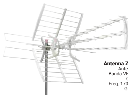
Antenna ZTL-368C05UV5G Antenna combo VU DDT, Banda VHF UHF, 20 elementi, Canali 6- 12 / 21- 48, Freq. 170-230 / 470-694 Mhz Guadagno VHF 10 dB UHF 12 - 15 dB
