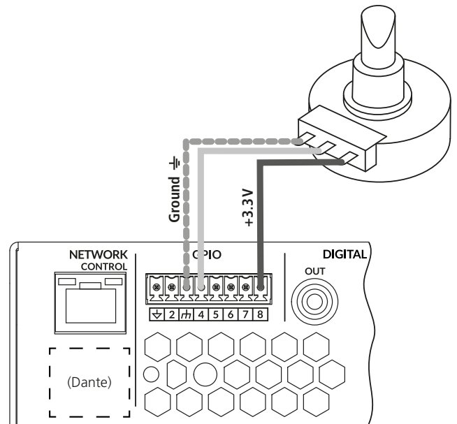
Abb. 10 externer Lautstärkereglер
