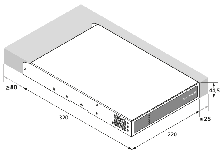
Abb. 4 Belüftungsabstände
