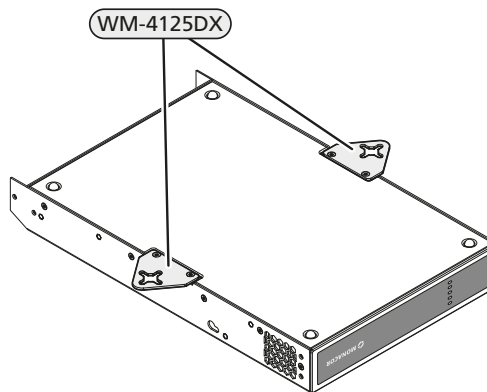
Abb. 8 Montageplatten an Geräteunterseite
