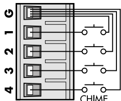
⑨ Branchement poussoir gong
