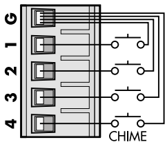
⑨ Anschluss Gongtaster
