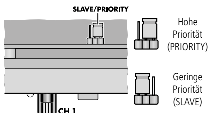
⑥ Wahl der Priorität eines Direkteingangs
