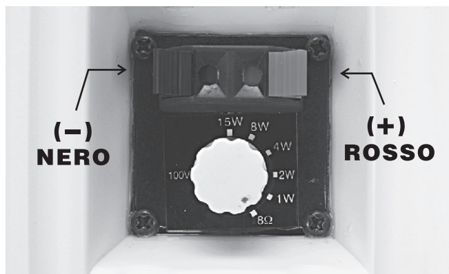
Terminali di collegamento
