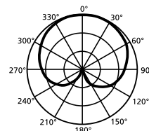
② Polardiagramm (bei 1 kHz) Polar pattern (at 1 kHz) Diagramme polaire (à 1 kHz)
