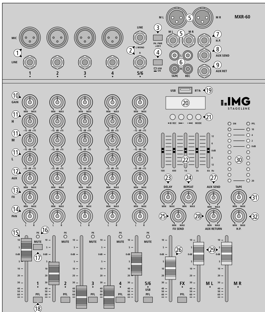
Abbildung MXR-60, bei den Modellen MXR-80/-120/-160 sind weitere Mono-Eingangskanäle vorhanden
