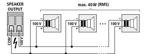
Abb. 2 Lautsprecheranschluss
